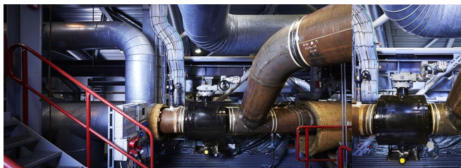
BROEN Ballomax® DN50 – podwójnie łożyskowany zawór z kulą jarzmioną, double block and bleed DBB, ze spustem w korpusie zaworu
